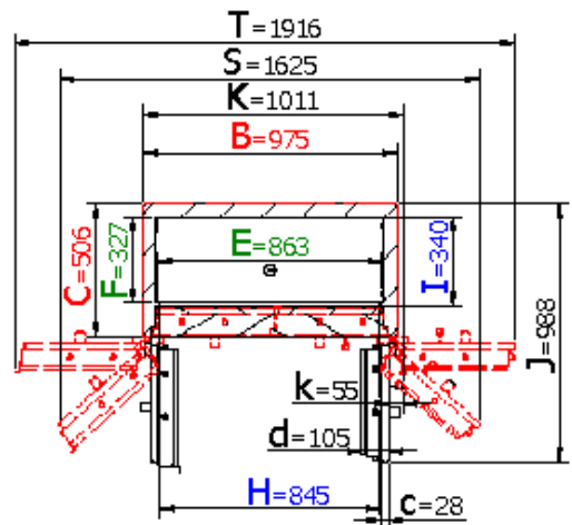
Draufsicht
