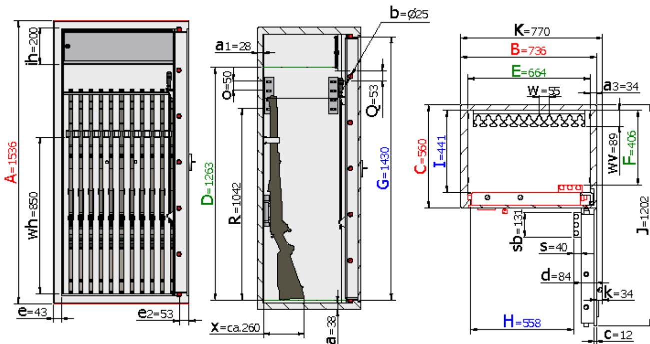
Frontalansicht
