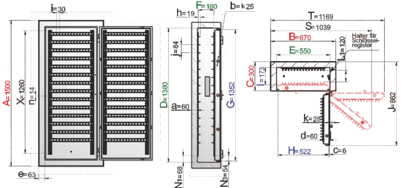
Frontansicht
