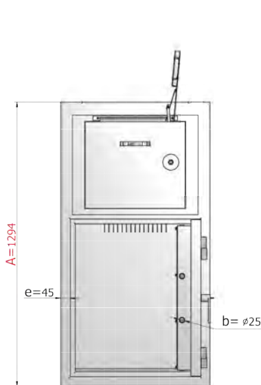
Frontansicht
