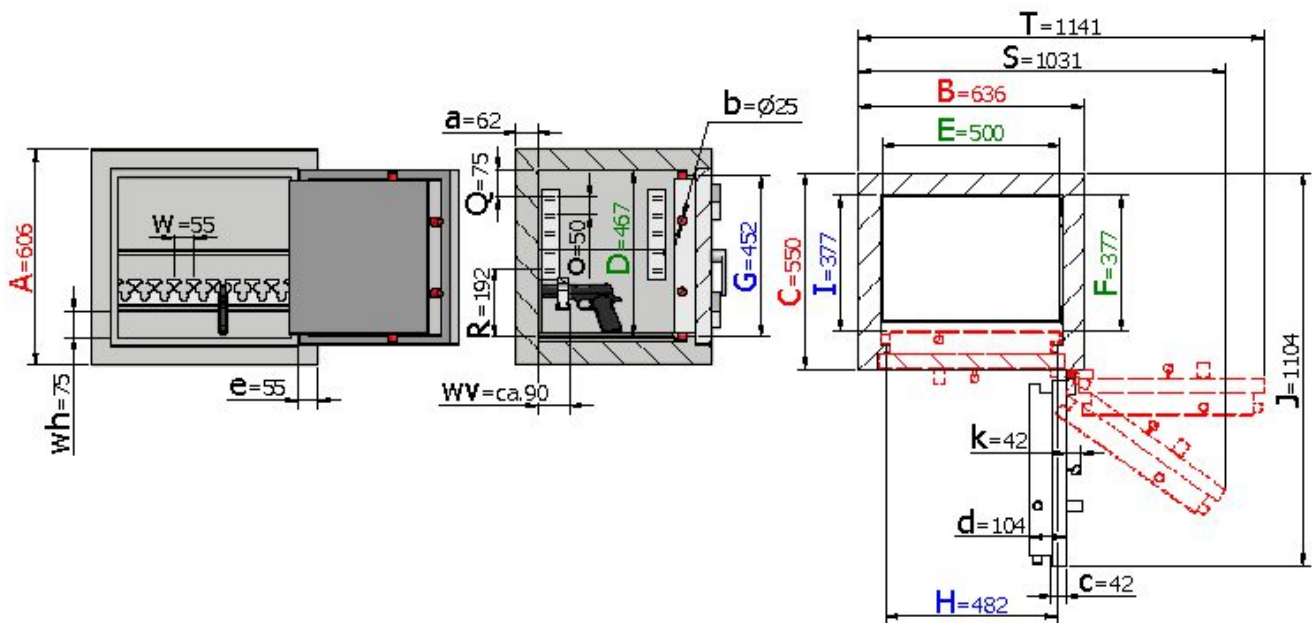
Frontalansicht
